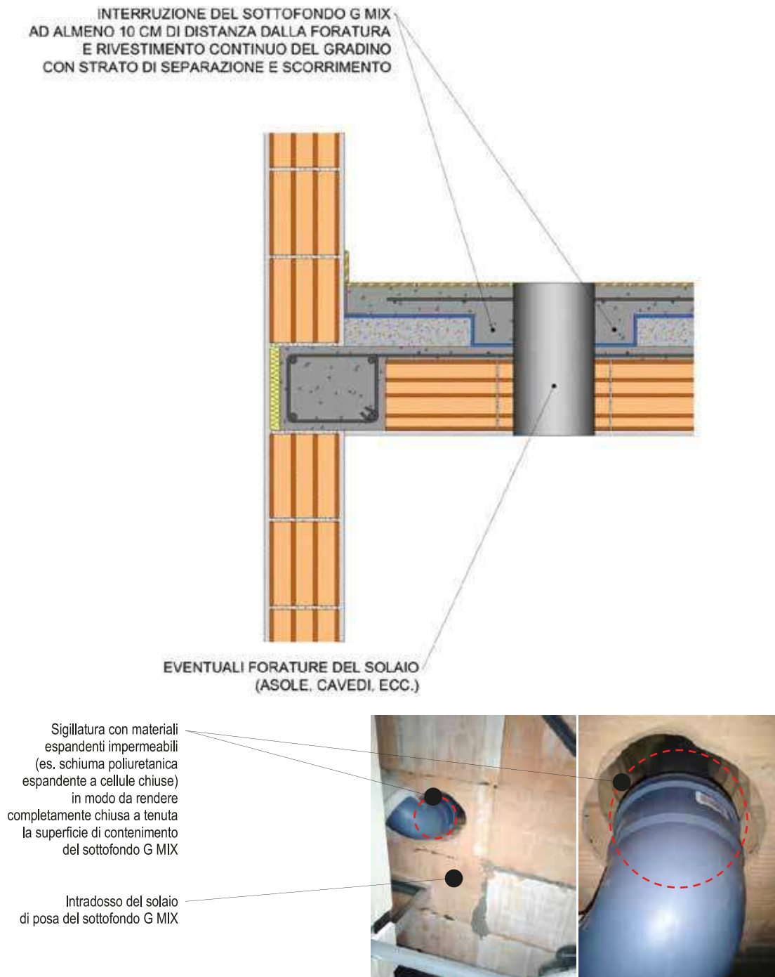
Particolari di posa FORATURE SOLAI
